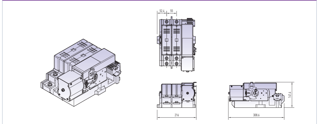
ATS-F TYPE [400A~600A] 3P 400AF
