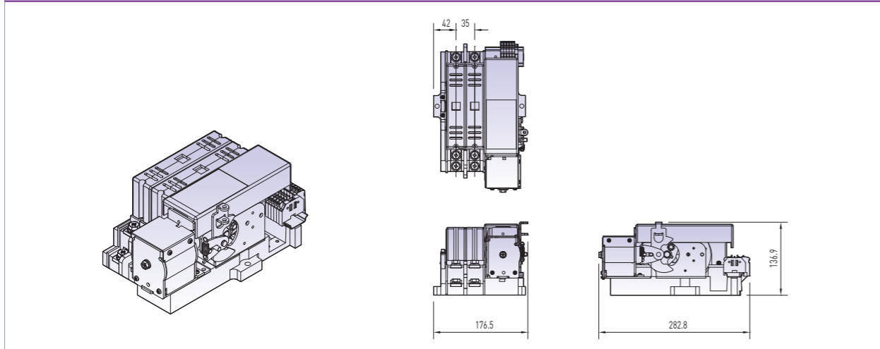
ATS-F TYPE [100A~200A] 3P 100AF
