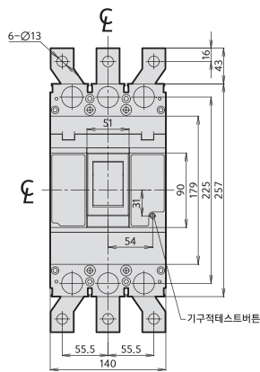
2, 3Pole
