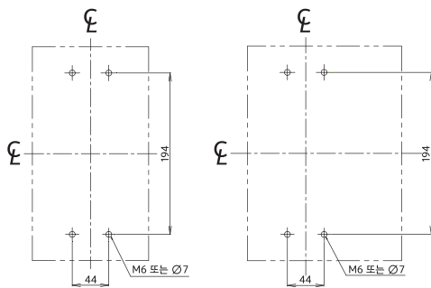
2, 3Pole
