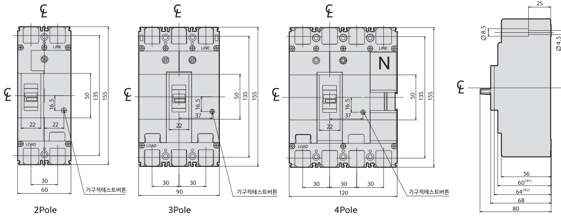
패널 설치치수
