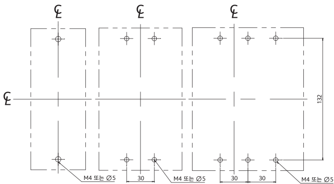
단자부 상세도
